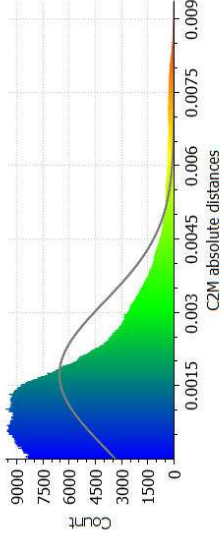
JPEG: 40
